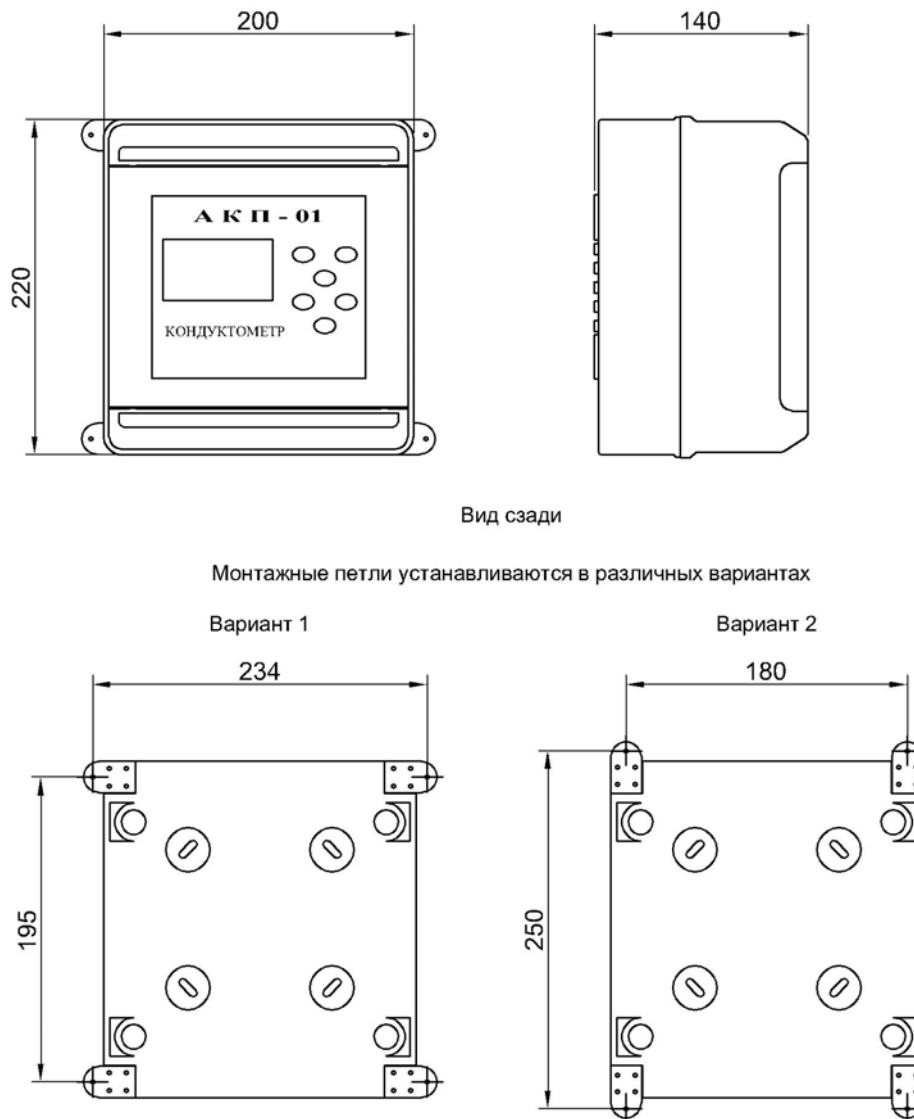
Рис. 2.2.1-1. Крепление ИУ
