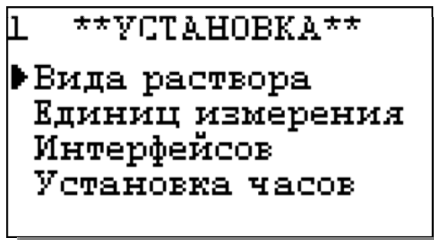
Рис. 2.3.3-2. Окно «УСТАНОВКА»
